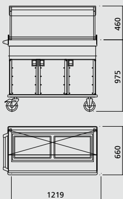
2xGN 1/1 quer
