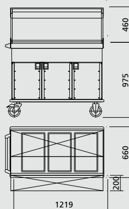
3xGN 1/1, 200 mm
